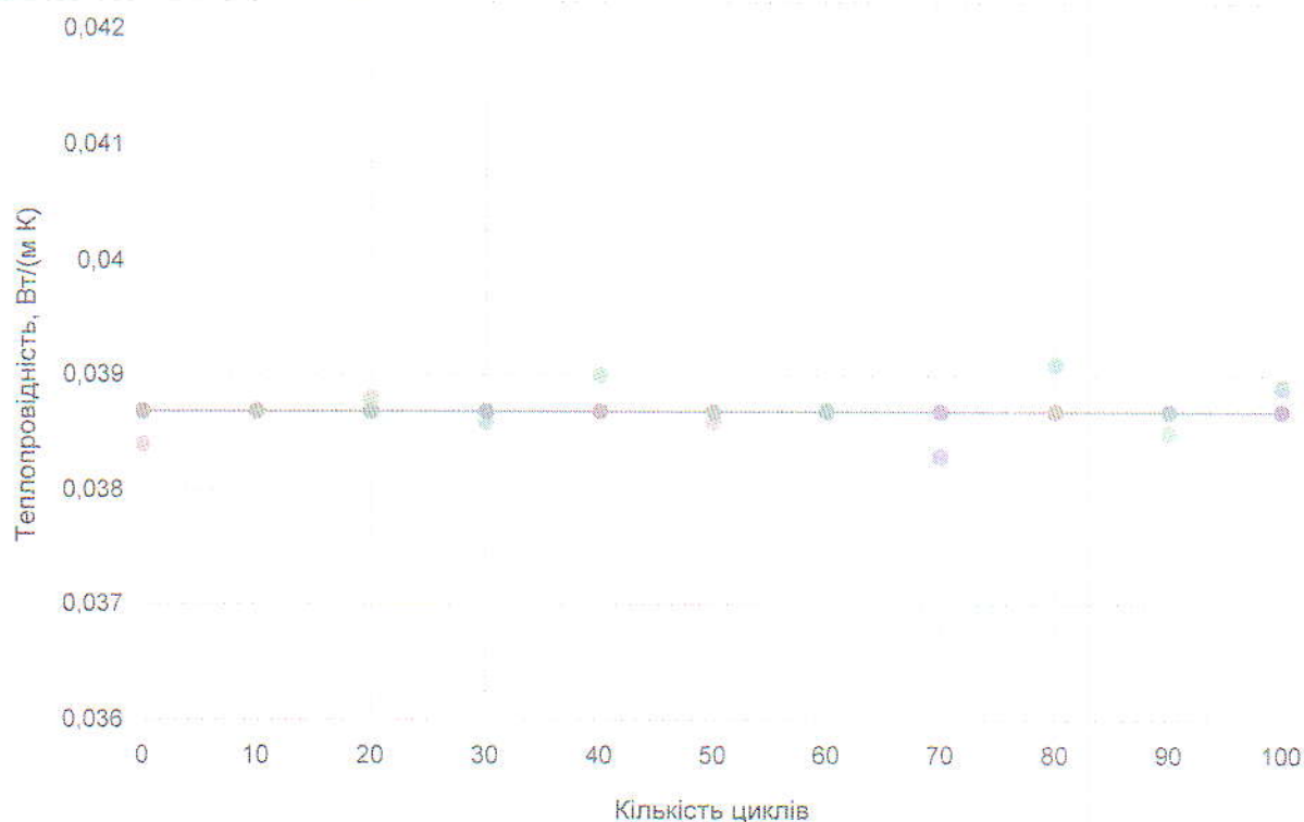
Рис.1 - Графік залежності теплопровідності матеріалу від кількості циклів.
